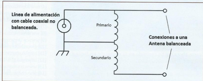
Imagen 2. Esquema eléctrico de un balun relación 4:1
