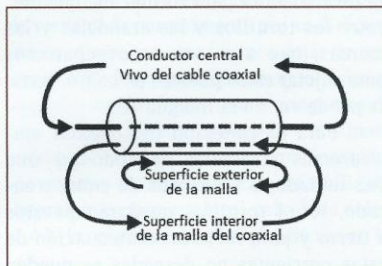
Imagen 5. Esquema de cómo fluyen las corrientes en un cable coaxial
