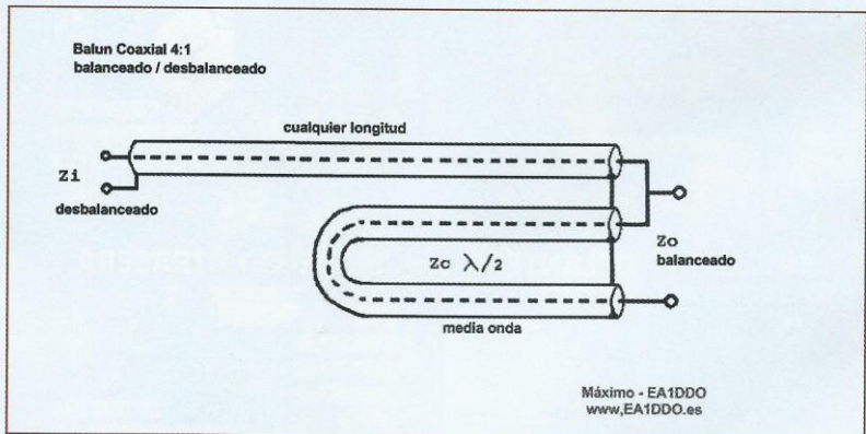
Imagen 3. Balun 4:1 realizado con cable coaxial
