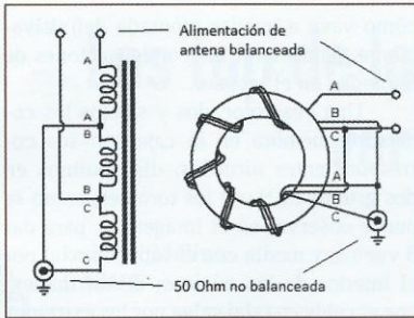
Imagen 4. Esquema de un balun 1:1 con núcleo de aire o de ferrita
