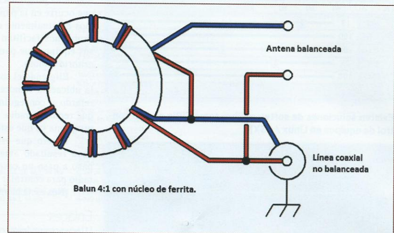
Imagen 1. Balun 4:1 con núcleo de ferrita
